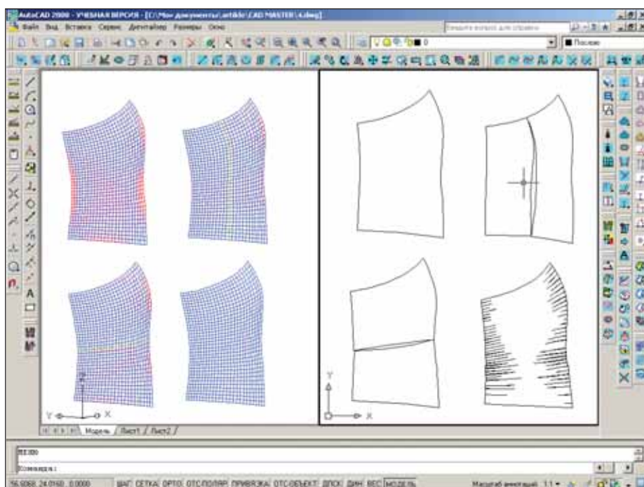
Варианты развертки боковой детали пиджака с различными параметрами алгоритма (показана визуализация деформаций при различных положениях разрезов и вариант развертки при условии полной нерастяжимости материала)
